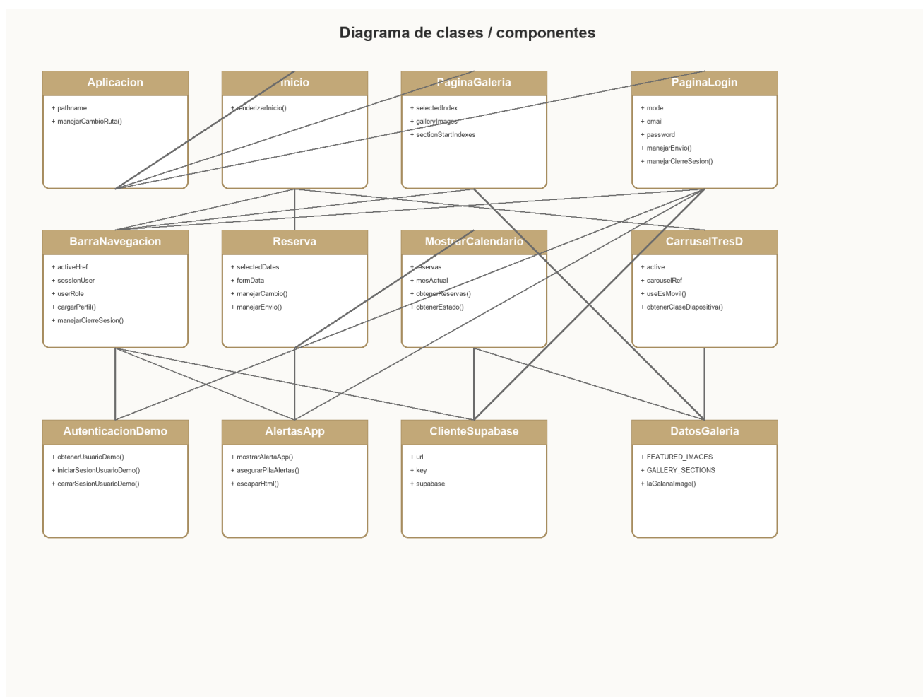
Figura. Diagrama de clases / componentes con nombres reales en español.
